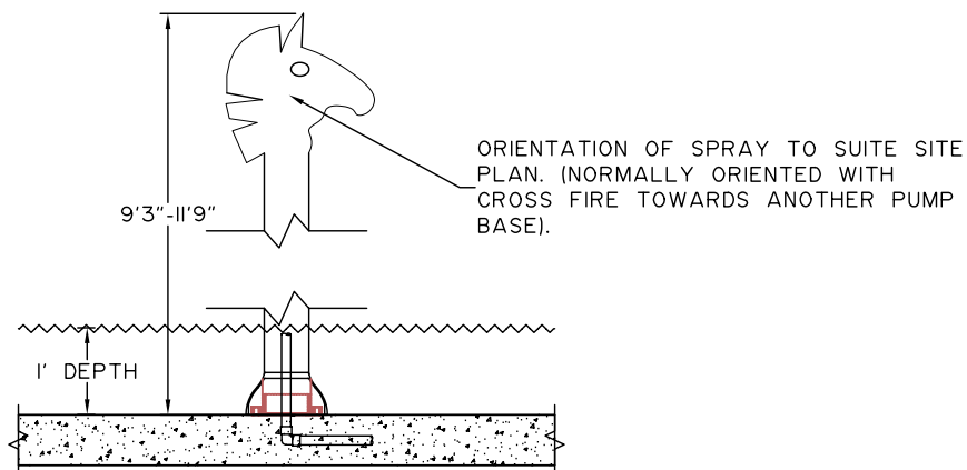
2 ELEVATION
